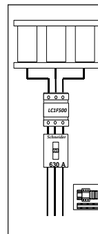
نمای تجهیزات پشت تابلو
